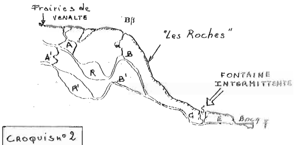
-- Schéma probable du mécanisme de la Fontaine intermittente de Crupet.
