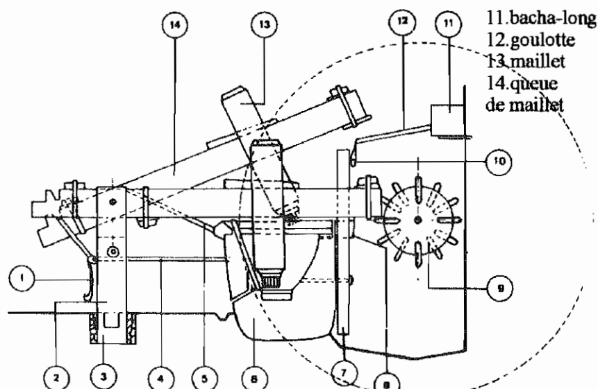
1. bêche 2. guide arrière 3. verge 4. bras de force 5. cheville longue 6. creux de pile 7. guide avant 8. bachalou 9. arbre à cames 10. couladou . . .
