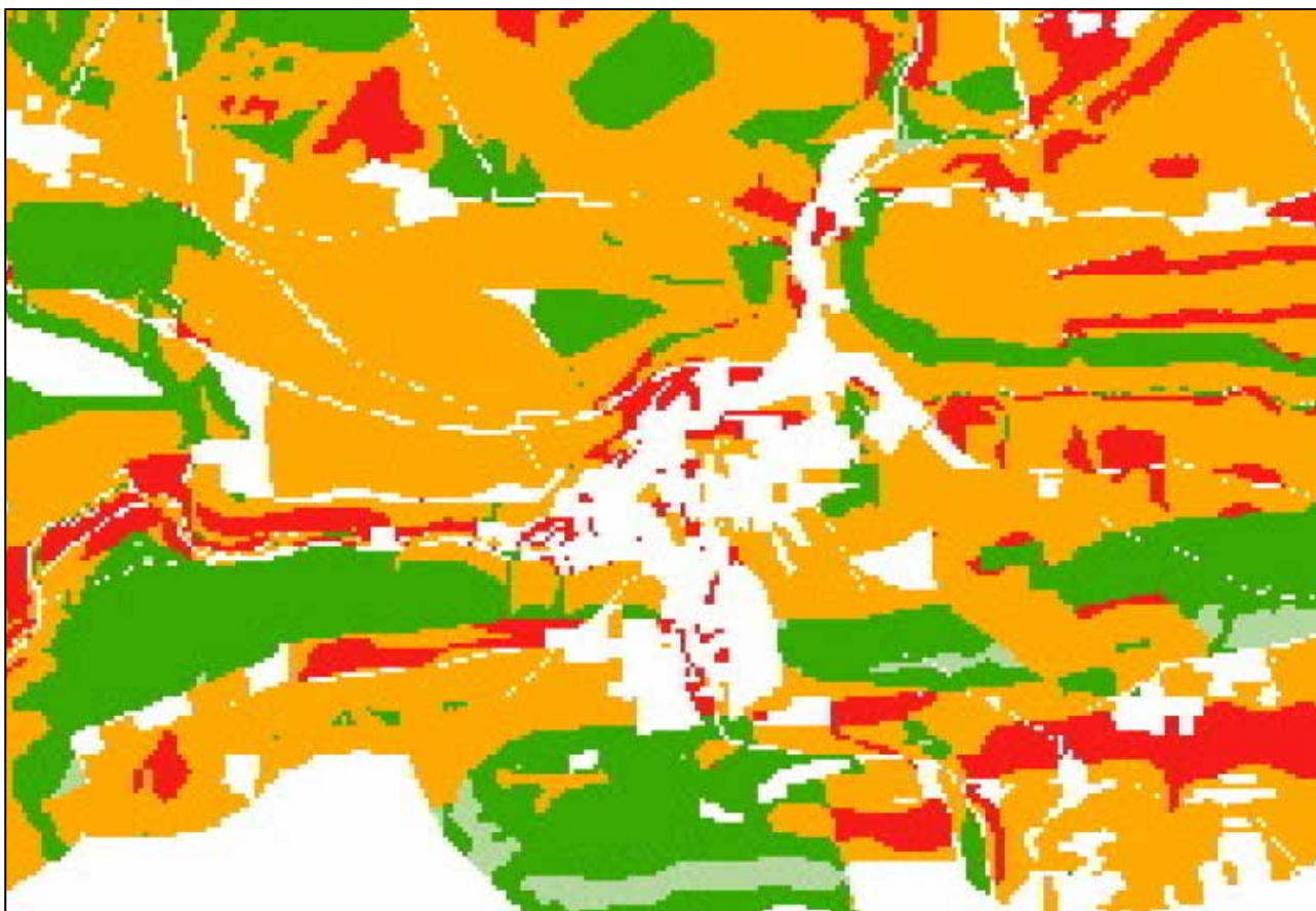
Carte de zones à risque de ruissellement diffus pour une pluie de 60mm durant une heure sur le bassin versant du Crupet (mémoire L. HIRTT, p. 20).
